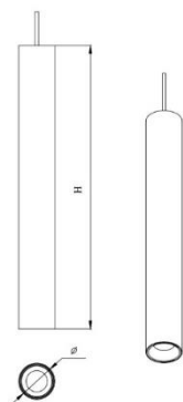
ГАБАРИТНЫЙ ЧЕРТЕЖ
